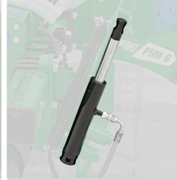
Koldan hidrolik markör sistemi: Her kolun bağımsız hareket etmesini sağlar. Hydraulic marker system: Provides each marker arm moving independently.
