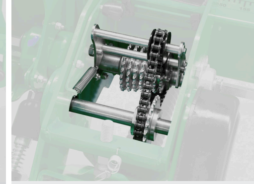
Tohum sıra üstü mesafesi ayar şanzımanı. Tohum ara mesafeleri dişli kutusudaki dişlilerin konumları tablo yardımıyla kolayca değiştirilerek yapılabilir. Seed in-line row distance adjustment transmission. Seed spacing is made easily by changing the positions of the gears in the gear box with the help of the indicator table.
